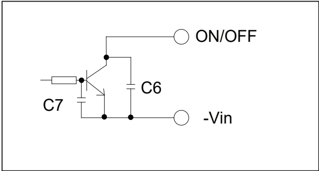
图 C: 晶体管控制方式
