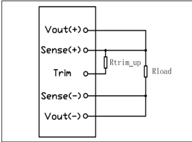
图 G: 输出电压上调示意图
